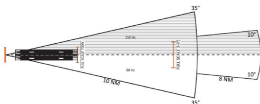
(a) Patrón emitido por el localizador (LOC).
