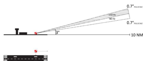
(b) Patrón emitido por la senda de planeo (GS).
